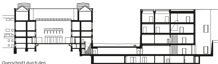
Querschnitt durch den Haupt- und Neubau
