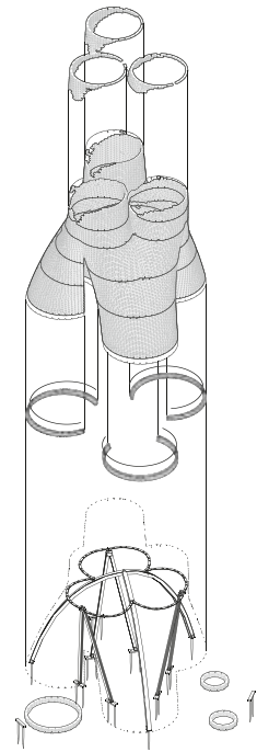
Konstruktionskonzept
